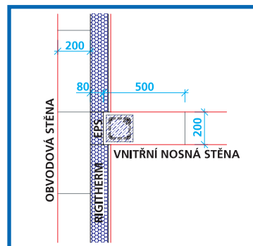
Obr. 5: Detail napojení nosné stěny
