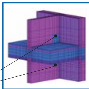
Obr. 6: Umístění ztraceného bednění
