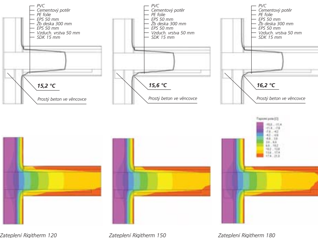
Obr. 4: Oblast kondenzace vodní páry v detailu
