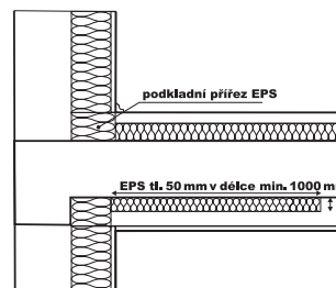
Obr. 2: Detail napojení stěny a stropu
