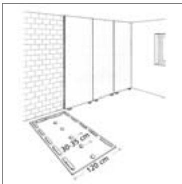
Obr. 8: Nanesení lepicího tmelu
