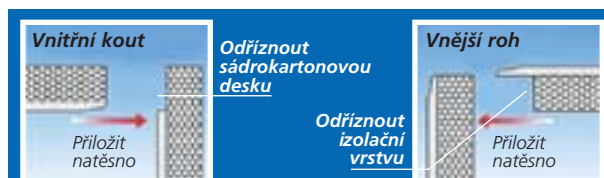
Obr. 9: Detail provedení nároží
